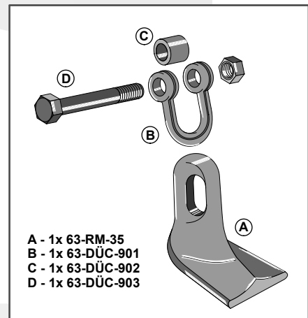
Ausführung mit Schäkel 54mm Modèle avec manille 54mm Model with shackle 54mm
