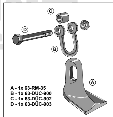
Ausführung mit Schäkel 66mm Modèle avec manille 66mm Model with shackle 66mm
